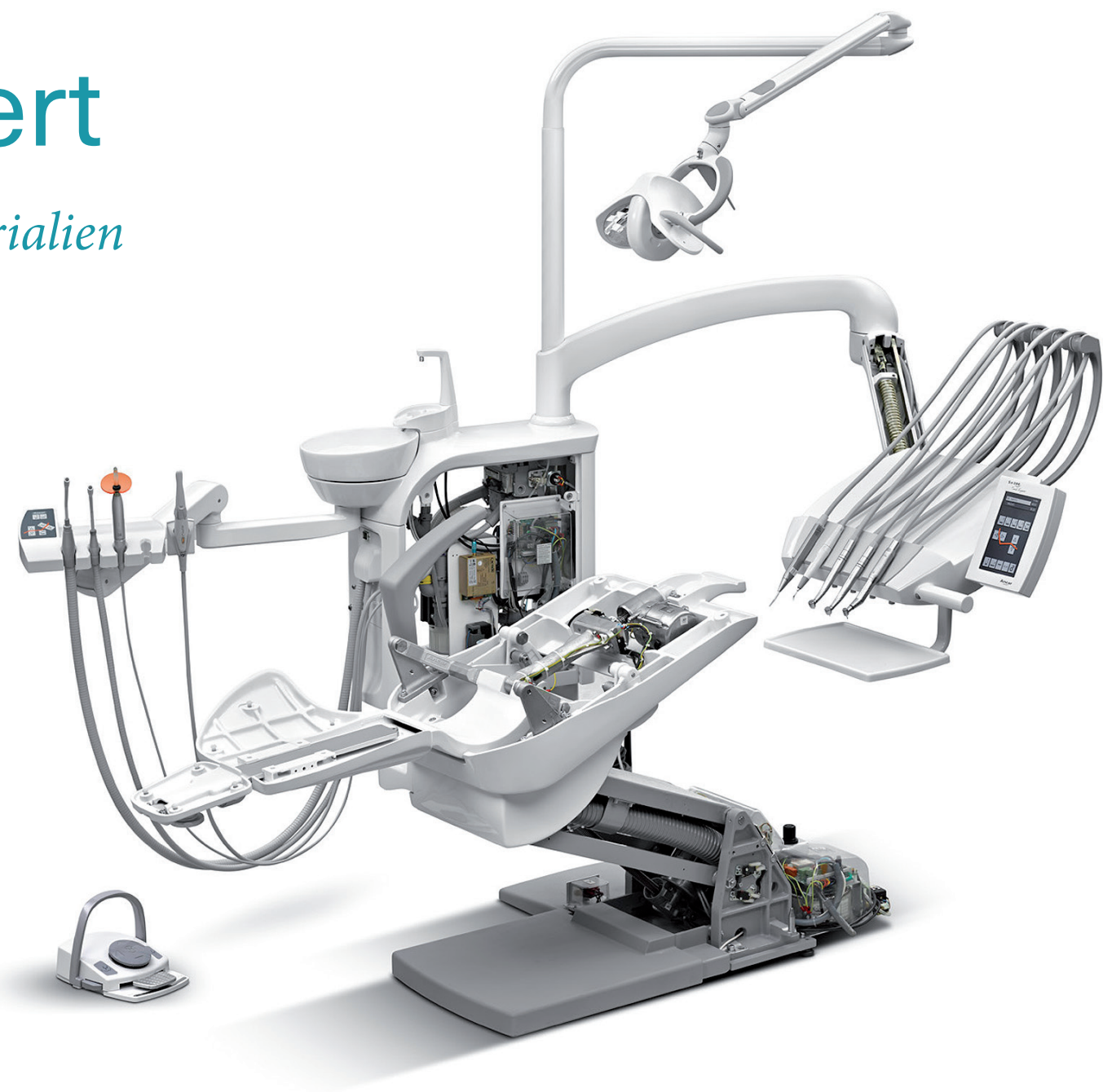
ALUMINIUMKERN alle tragenden Teile der Einheit
